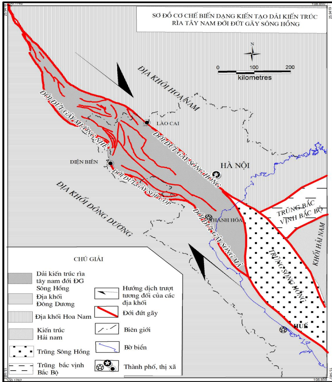
Hình 3. Sơ đồ cơ chế biến dạng kiến tạo Kainozoi muộn dải kiến trúc rìa tây nam đối đứt gãy Sông Hồng,
